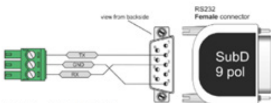
Abb.1 Spezial RS232-Kabel
